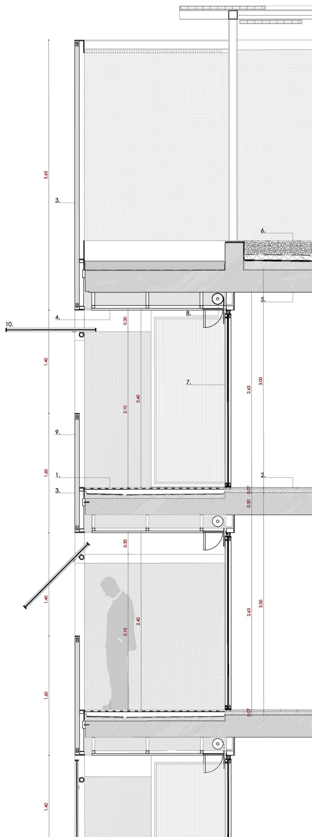
DETALL CONSTRUCTIU escala 1/25
