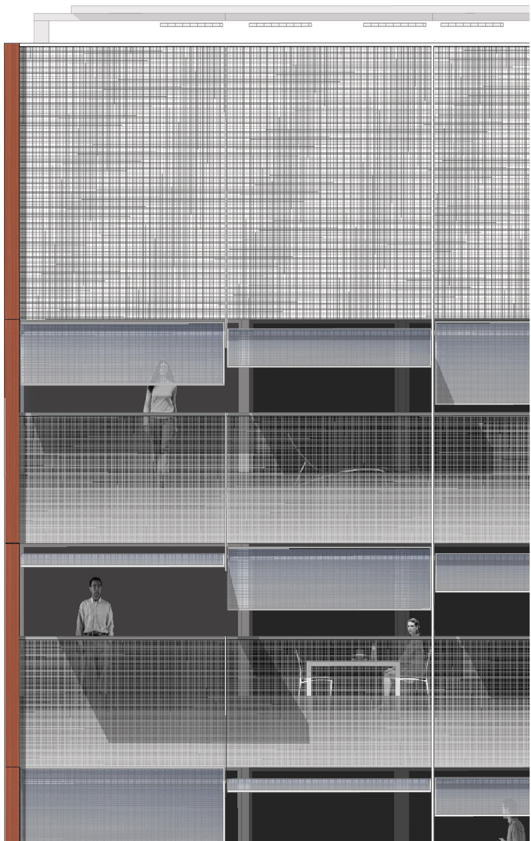
IMATGES DIA I NIT DETALL ALÇAT escala 1/25
